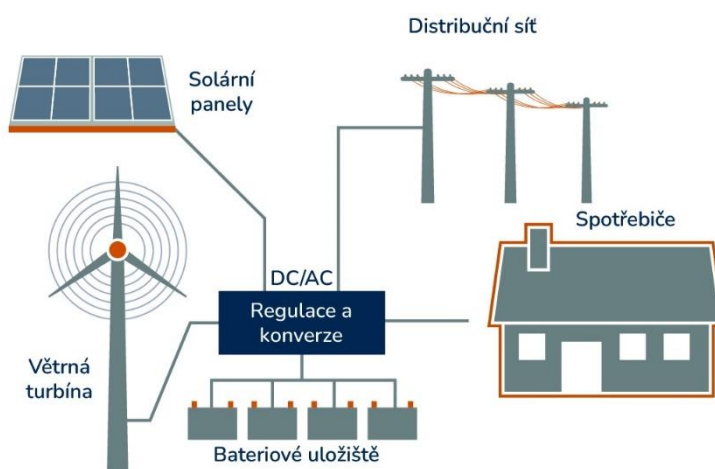
Obrázek 58: V řadě případů VtE přímo na budovách nemá smysl, variantou je menší VtE na stožáru, kombinovaný systém VtE s FVE vč. akumulace. Schéma, vlastní zpracování.
