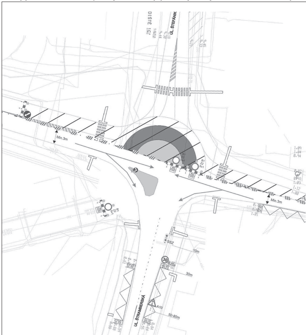
Řidiči se musejí připravit na dopravní omezení vyznačená na plánu. Budování kruhového objezdu v místě křižovatky u Kachlovky bude znamenat další komplikace na silnicích. REPRO: MĚSTO KOPŘIVNICE
